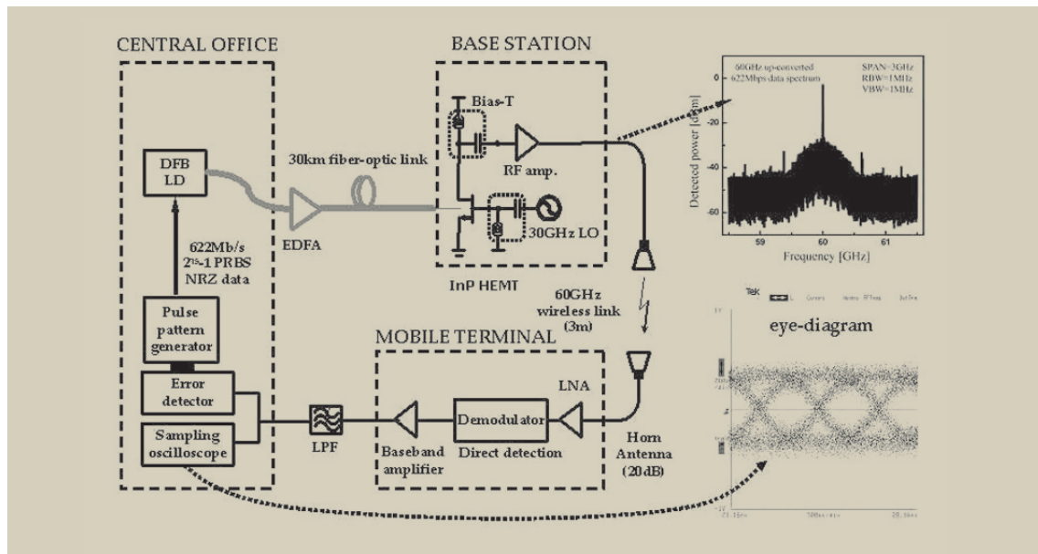
그림 6. HEMT 광전 주파수 변환기를 사용한 60GHz 대역 RoF 하향 전송
