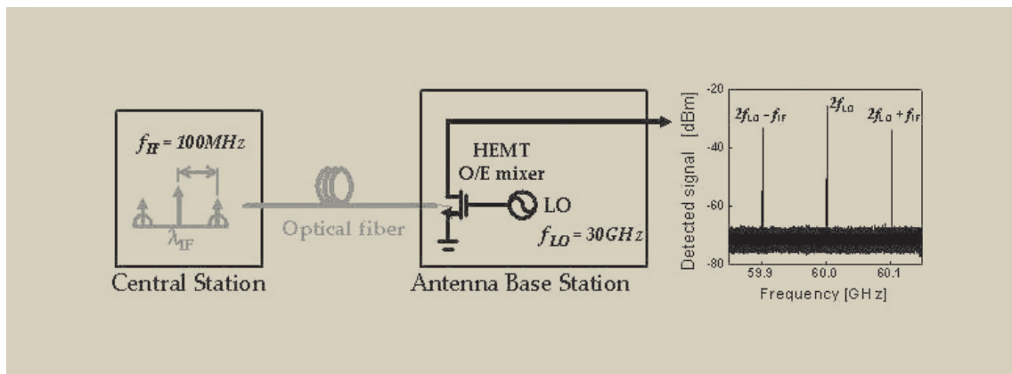
그림 5. HEMT 광전 주파수 변환기를 사용한 RoF 시스템
