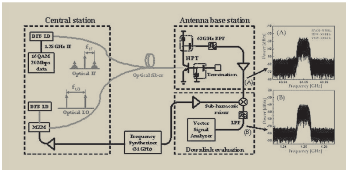
그림 8. HBT 광전 주파수 변환기를 이용한 60GHz 대역 RoF 하향 전송
