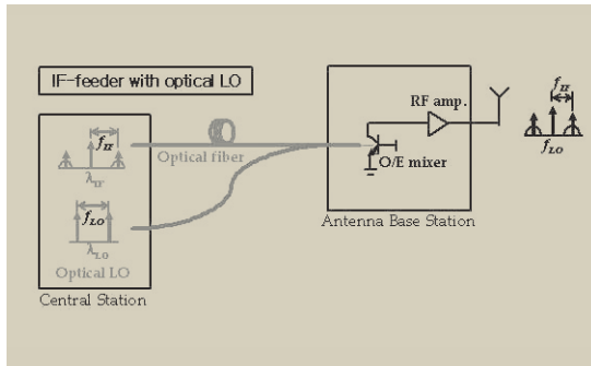
그림 7. 광학적 LO를 사용하는 IF-feeder 방식의 RoF 시스템
