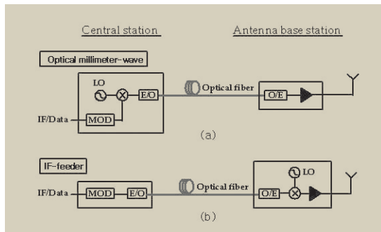
그림 2. RoF 시스템의 구성도
