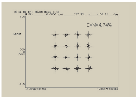
그림 13. 복원된 16QAM 신호의 constellation 및 EVM
