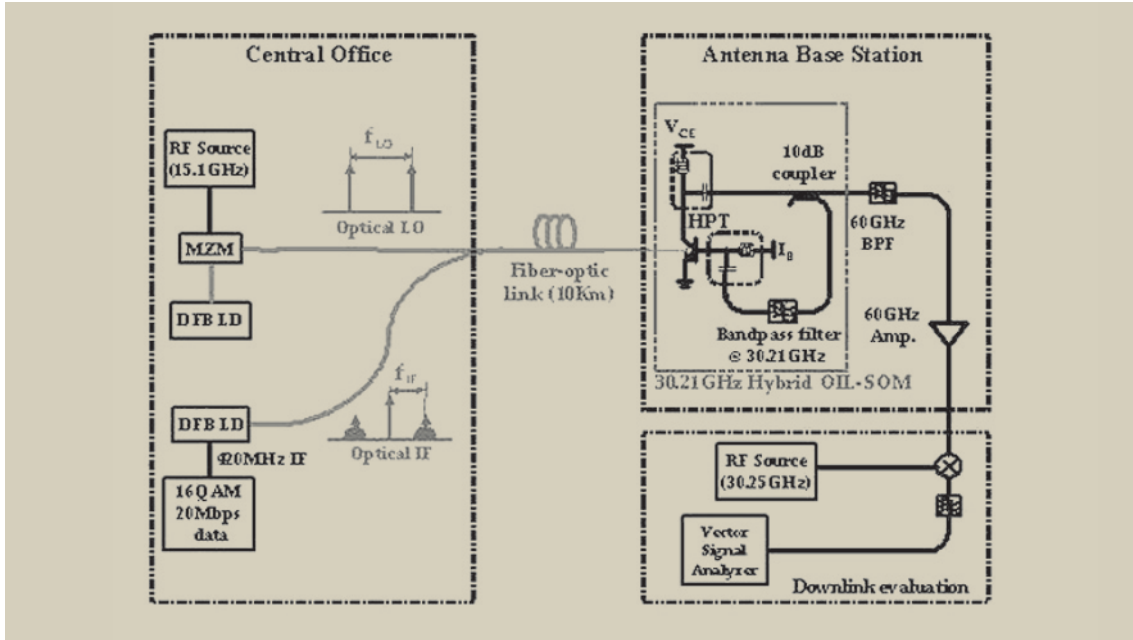
그림 10. HBT OIL-SOM을 이용한 60GHz RoF 하향 전송 시스템
