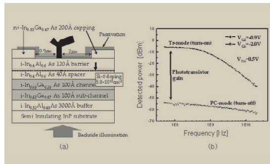
그림 3. InP HEMT의 (a)적층구조와 (b)측정된 광변조 응답
