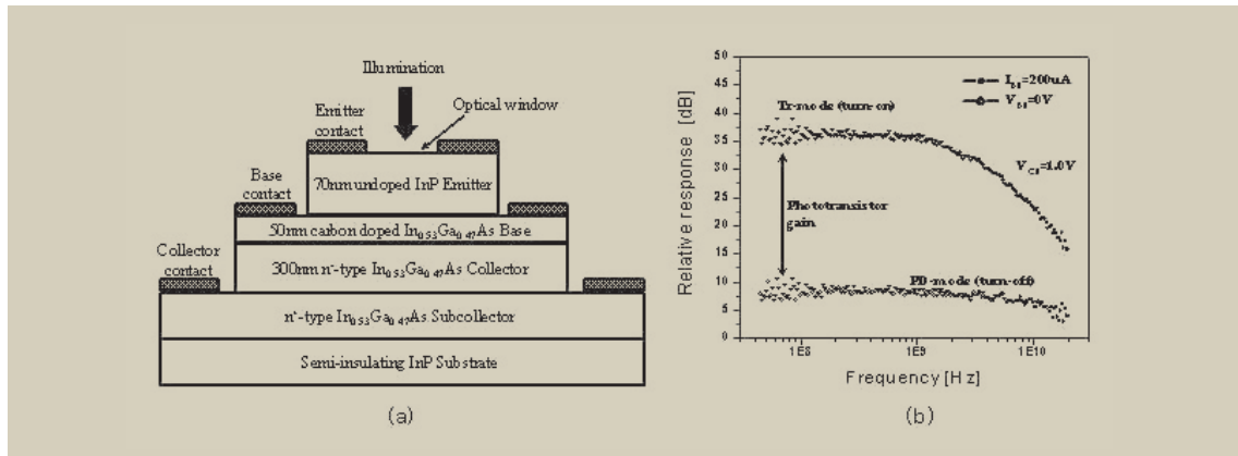
그림 4. InP HBT의 (a)적층구조와 (b)측정된 광변조 응답
