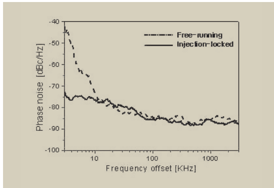
그림 11. free-running 및 위상 고정 발진기의 위상 잡음
