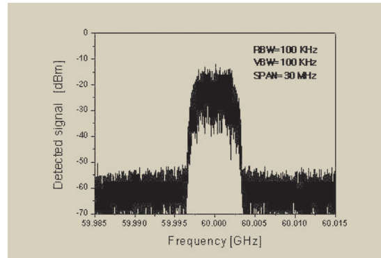
그림 12. 주파수 상향 변환된 신호의 RF 스펙트럼
