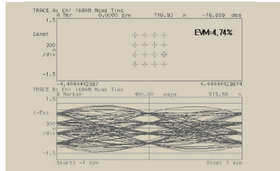
그림 9. 복원된 16QAM 신호의 constellation 과 eye-diagram
